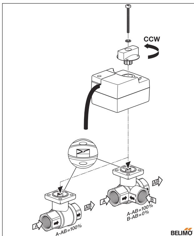
Kuva 1: Venttiili ja toimilaite avautuvat vastapäivään ja sulkeutuvat myötäpäivään. Kuvassa venttiili ja toimilaite ovat täysin auki. Näkyvissä on myös nesteen sallittu virtaussuunta.
