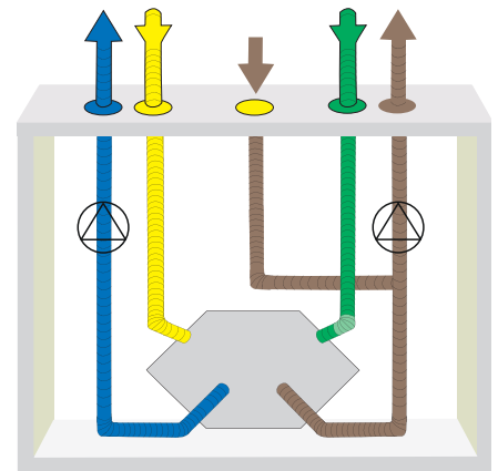
CASA W4 Smart XS R, oikeakätinen versio
