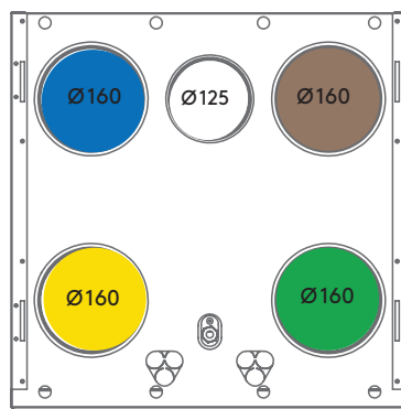
CASA W4 Smart XS R, oikeakätinen versio
