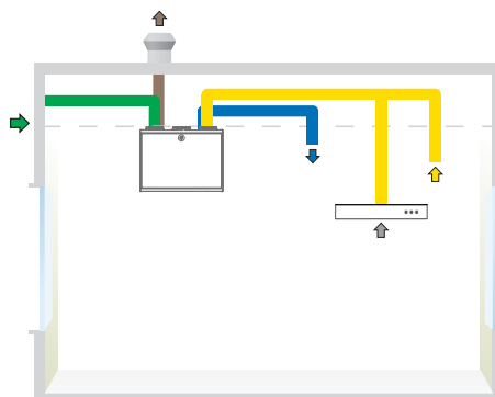
CASA W4 Smart xs L kanavaliitännät ja liesikupu liitettynä poistoilmakanavaan.
