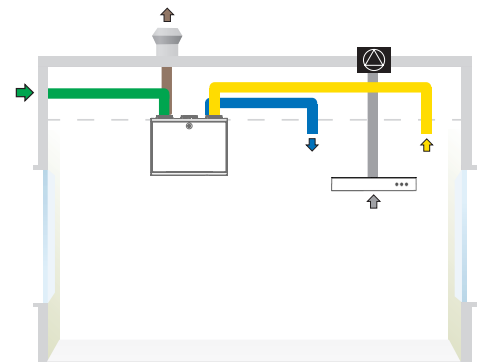
CASA W4 Smart xs L kanavaliitännät ja liesikupu liitettynä ulkoiseen huippu- imuriin.
