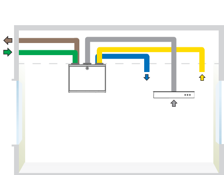
CASA W4 Smart xs L kanavaliitännät ja liesikupu liitettynä ilmanvaihdon keittiökanavayhteeseen.
