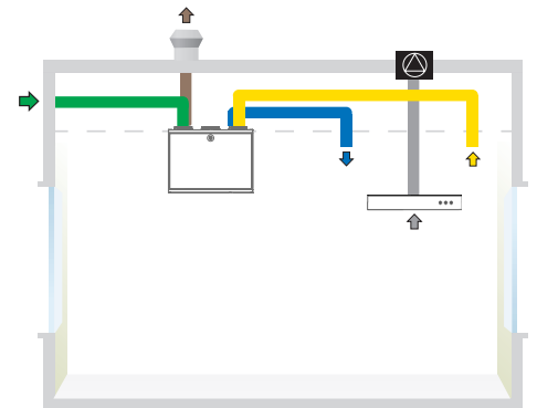
CASA W3 Smart xs L kanavaliitännät ja liesikupu liitettynä ulkoiseen huippu- imuriin.
