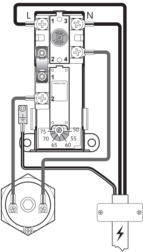
Электроподключение, схема
