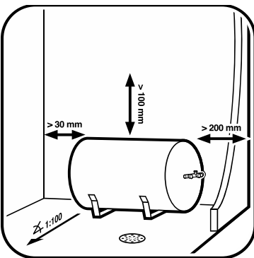
Kuva 5. VLS-tuotteen asennus.
