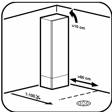
Kuva 4. Asennuksen suojaetäisyydet.
