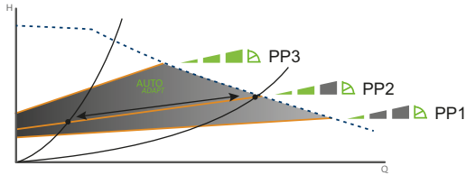
Kuva 15 Kolme suhteellista painekäyrää
