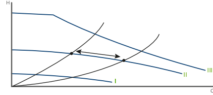
Kuva 17 Kolme vakiokäyrä-/vakionopeusasetusta
