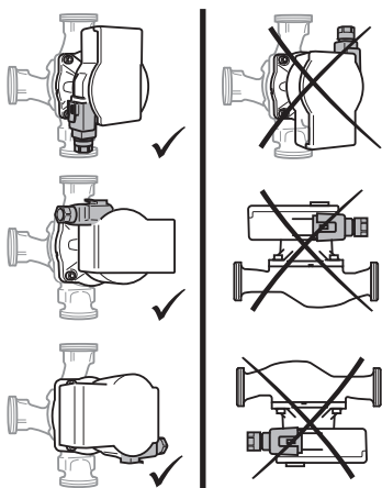
Fig. 2: Asennusasennot
